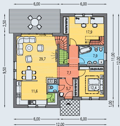
PRÍZEMIE [plocha 102.0 m 2 ]
