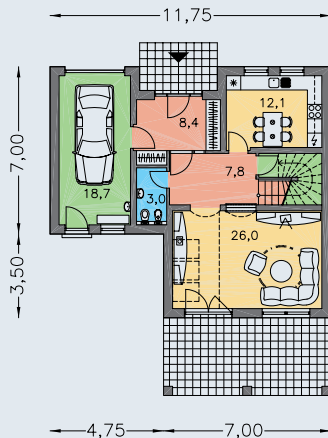
PRÍZEMIE [plocha 83.0 m 2 ]
