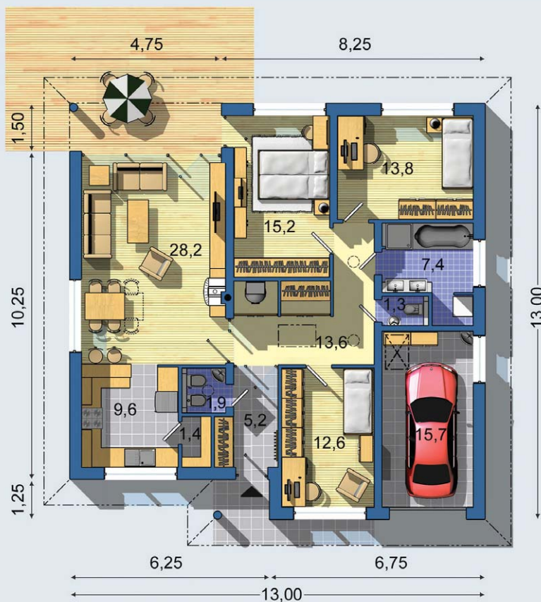
PRÍZEMIE [celková plocha 125.9 m 2 ]
