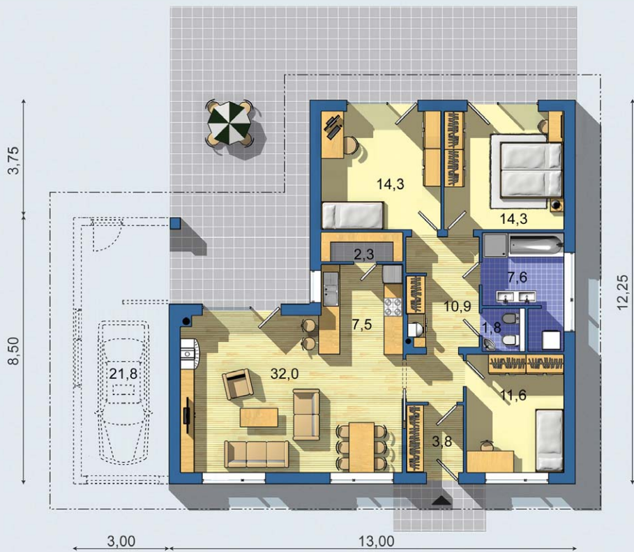
PRÍZEMIE [celková plocha 106.2 m 2 ]
