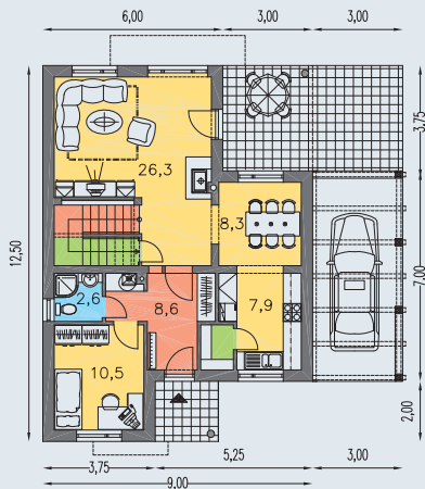
PRÍZEMIE [plocha 74.0 m 2 ]
