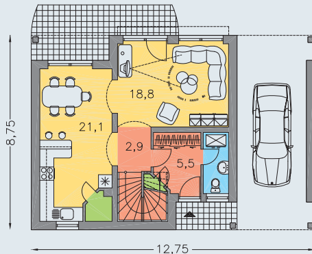
PRÍZEMIE [plocha 59.8 m 2 ]
