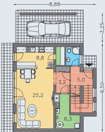
PRÍZEMIE [plocha 62.0 m 2 ]
