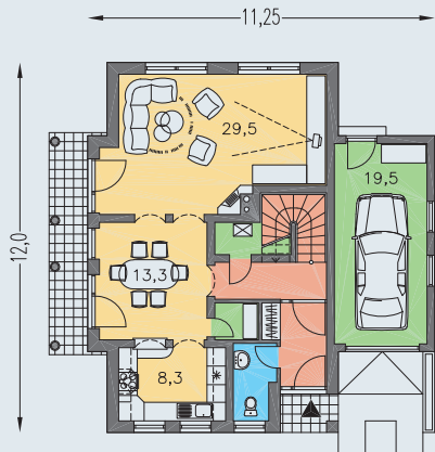
PRÍZEMIE [plocha 94.3 m 2 ]
