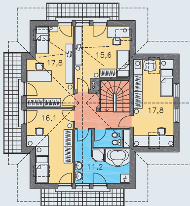
POSCHODIE [plocha 111.2 m 2 ]
