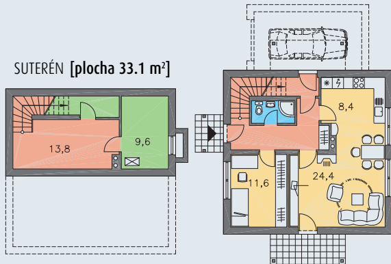
PRÍZEMIE [plocha 62.1 m 2 ]
