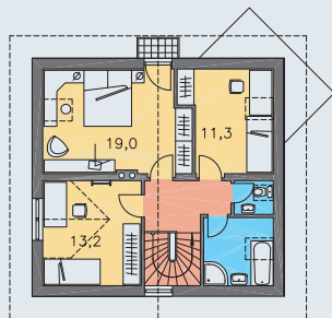
POSCHODIE [plocha 57.3 m 2 ]
