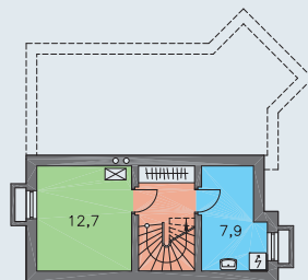
SUTERÉN [plocha 30.1 m 2 ]
