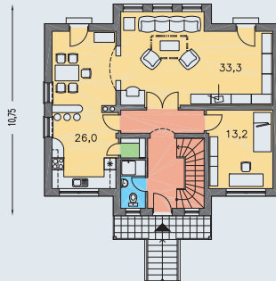
PRÍZEMIE [plocha 83.2 m 2 ]
