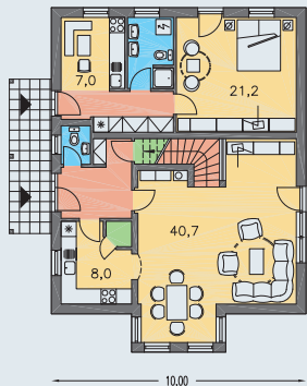
PRÍZEMIE [plocha 100.5 m 2 ]
