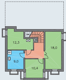
SUTERÉN [plocha 60.5 m 2 ]
