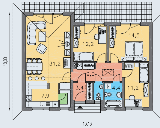
PRÍZEMIE [plocha 97.2 m 2 ]
