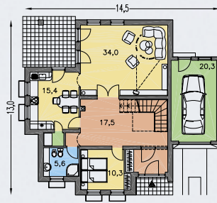
PRÍZEMIE [plocha 117.5 m 2 ]
