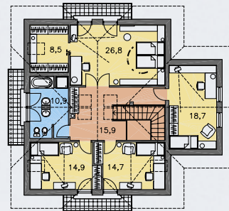
POSCHODIE [plocha 126.8 m 2 ]
