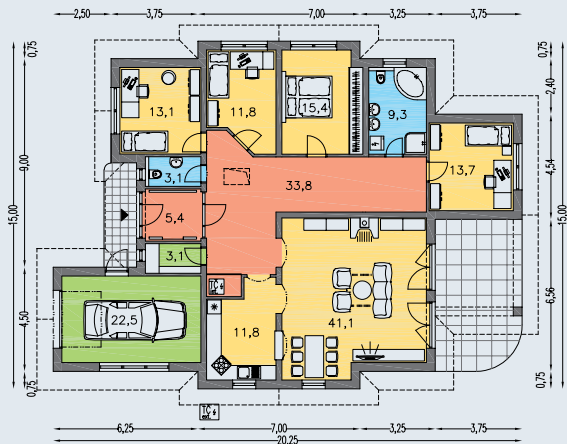
PRÍZEMIE [plocha 183.9 m 2 ]
