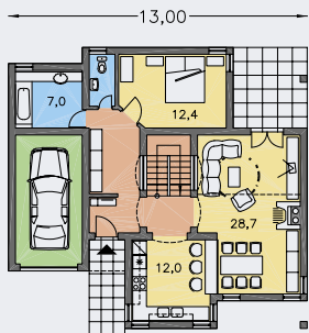
PRÍZEMIE [plocha 97.2 m 2 ]
