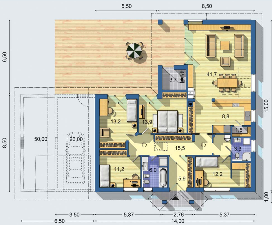
PRÍZEMIE [celková plocha 136.8 m 2 ]
