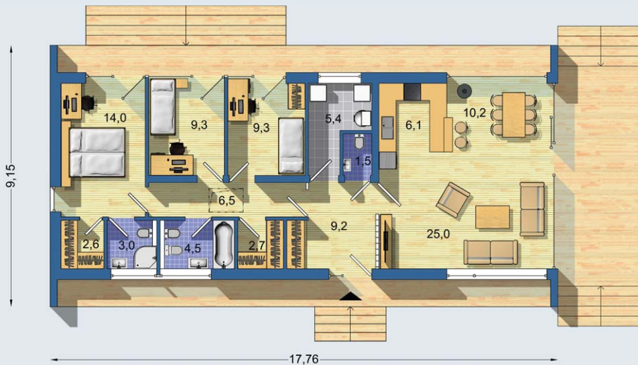
PRÍZEMIE [celková plocha 109.3 m 2 ]
